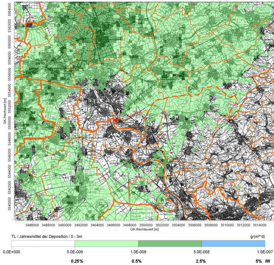
Bild A-11: Thallium-Deposition Jahresmittelwert (Rechengebiet)
