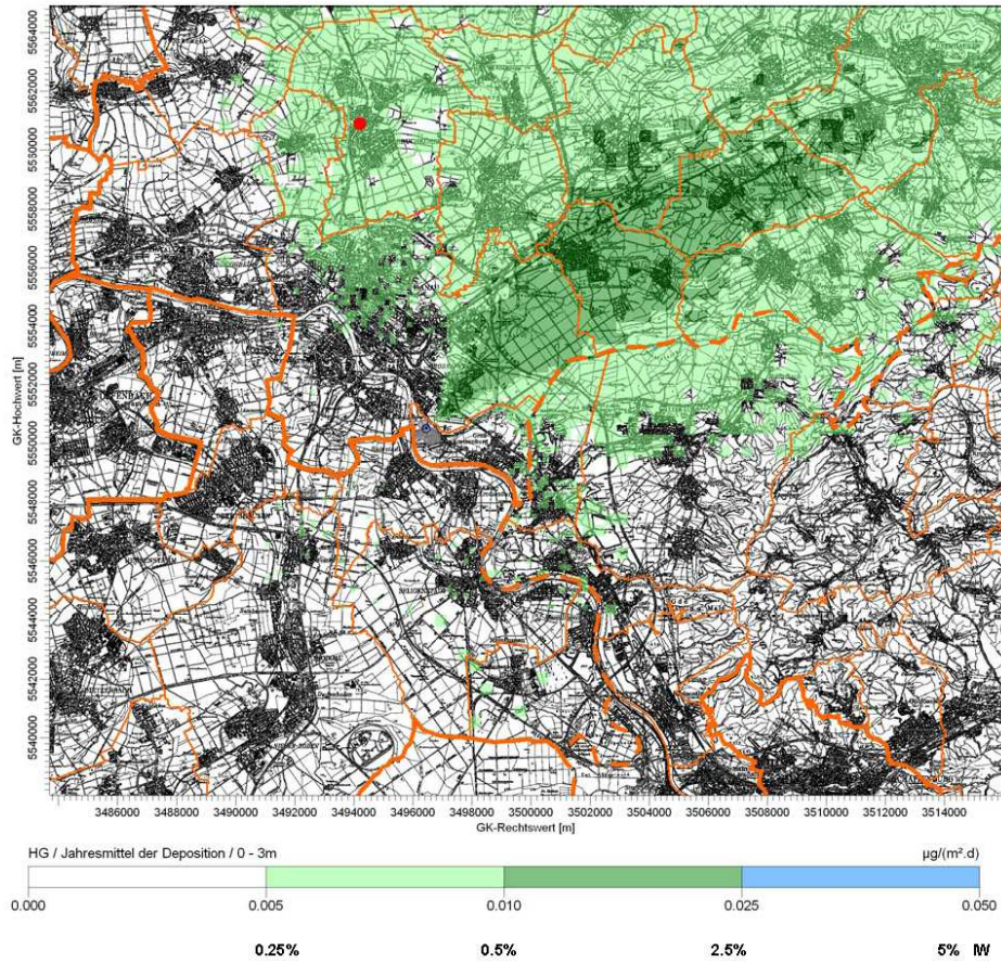
Bild A-10: Quecksilber-Deposition Jahresmittelwert (Rechengebiet)
