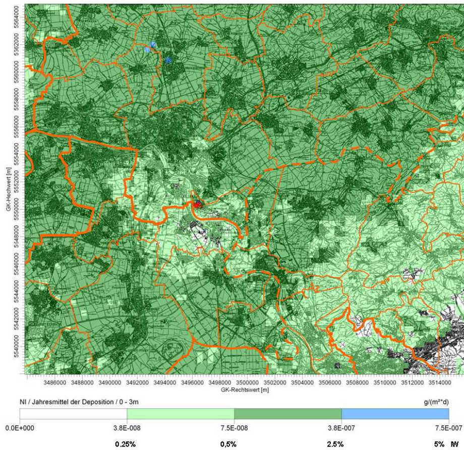
Bild A-9: Nickel-Deposition Jahresmittelwert (Rechengebiet)
